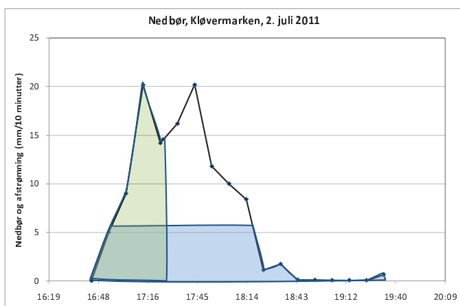
Figur 1. Kloakker håndterer de blå vandmængder ved at sende dem videre til rensesanlæg, vandløb og havet, mens LAR-anlæg håndterer de grønne vandmængder ved at holde dem tilbage i lokalområderne. Linjerne er angivet for hhv. et LAR-anlæg med lille nedsivningskapacitet og for et kloaksystem for et meget stort opland.
